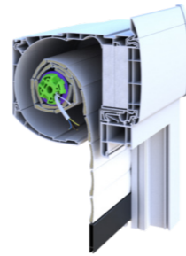
Coffre extérieur CRX
