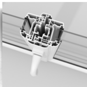
Masse centrale 114 mm
