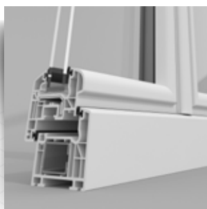
Ouvrant affleurant de 80 mm
